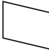
rhombus
